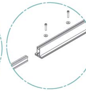
EINZELHEIT C
