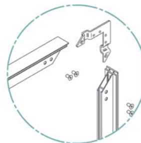
EINZELHEIT A
